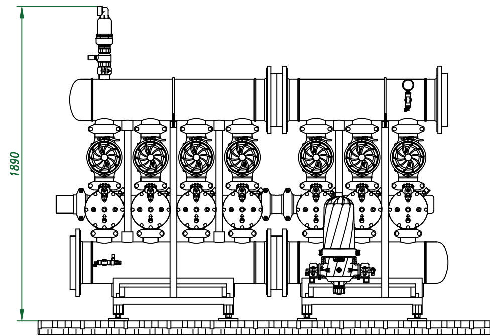
Вид спереди
